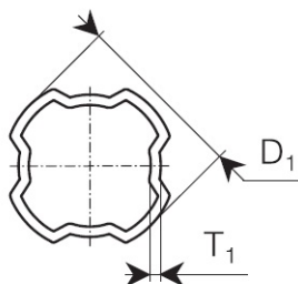
Внешняя труба
