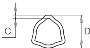
Внутренняя труба
